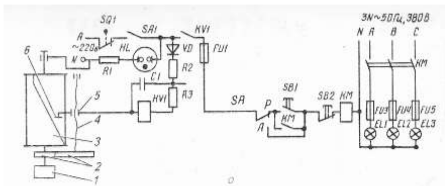
Рис. 1. Принципиальная электрическая схема освещения птичников УПУС -1.
